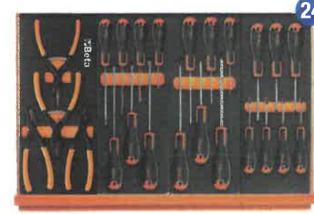
M145 M214 M216 M217
